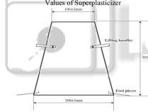
Fig. 1: Slump Cone Apparatus
